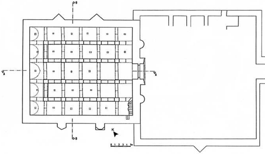
Çizim 1: Denizli Çardak Han Rölöve Planı 30
